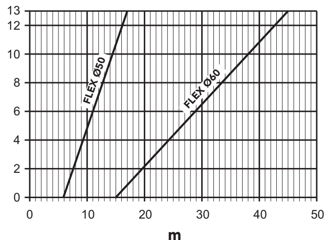
fig. 27 - Grafico per scelta parametro camino
