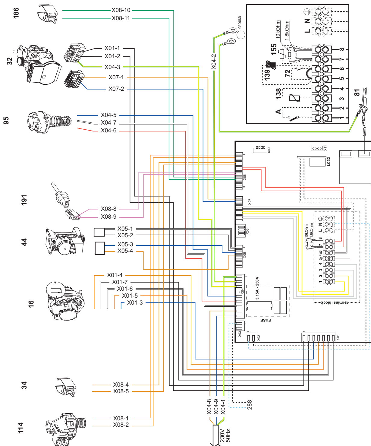
рис. 58- Электрическая схема
